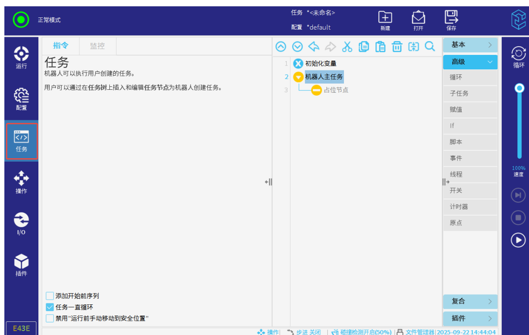
图 3-98: 任务选项卡
