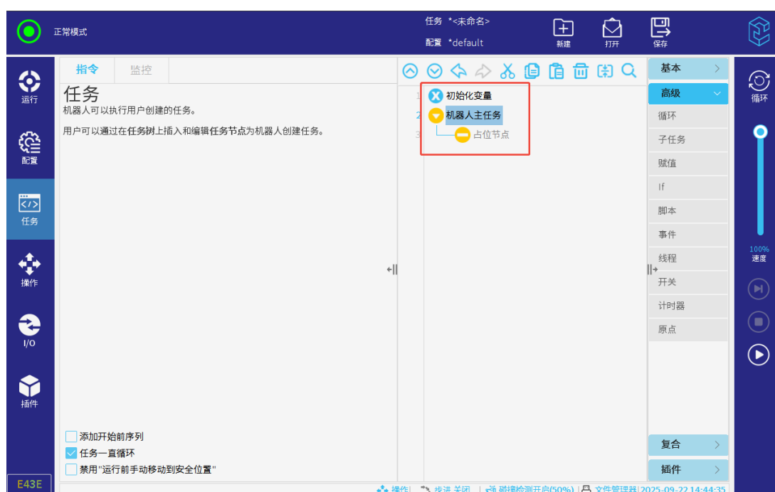
图 3-99: 任务树
