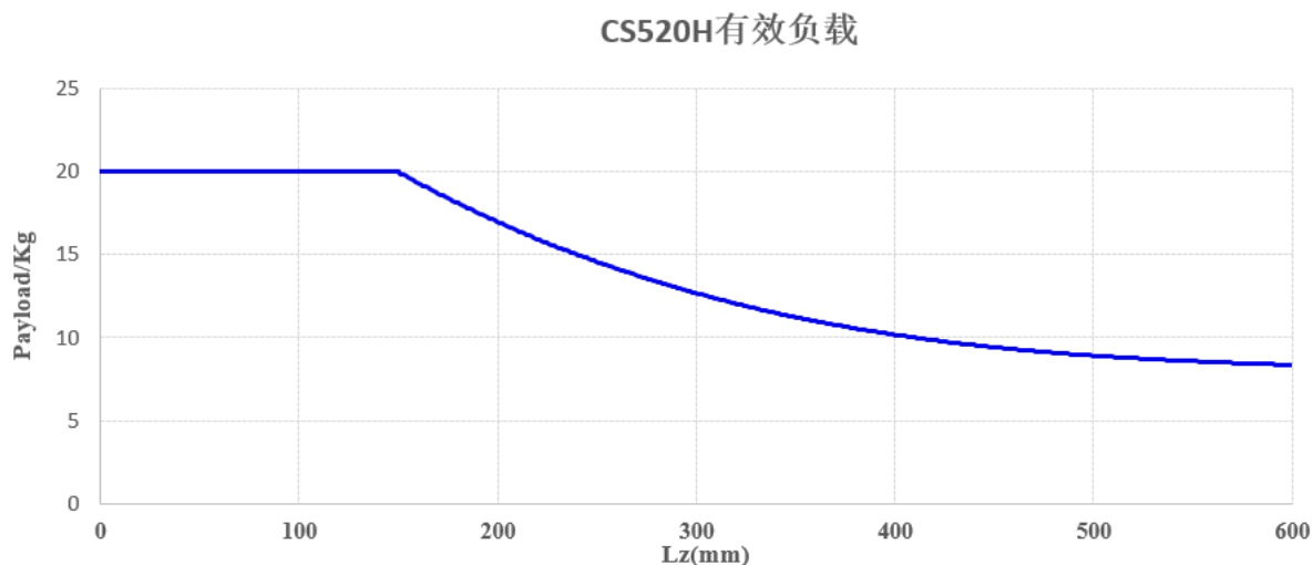
图 2-7: 有效负载图
