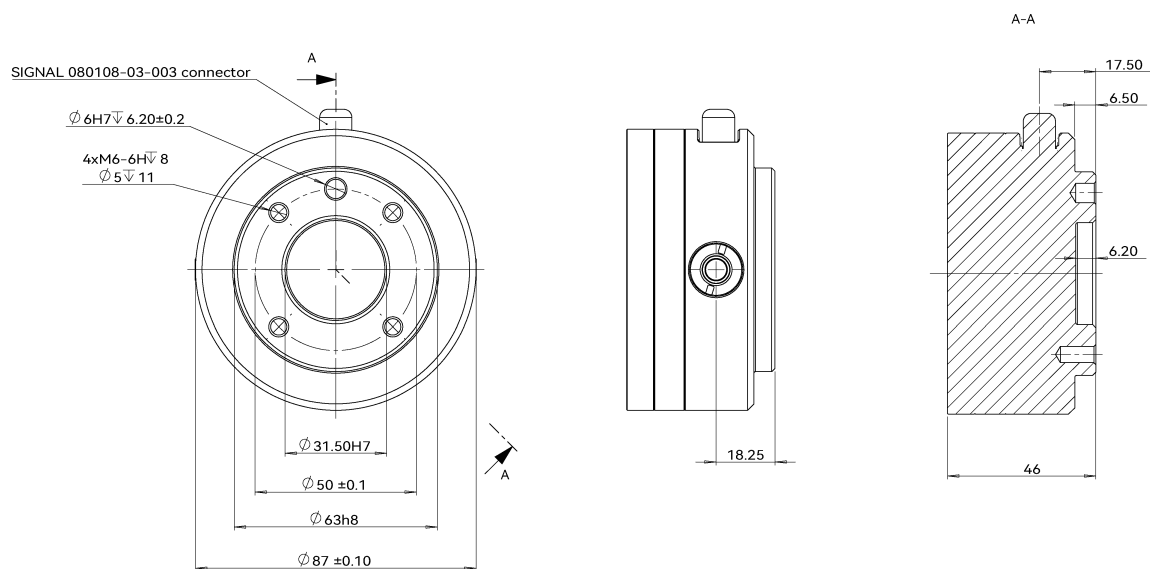
图 2-5: CS520H 机器人工具法兰安装尺寸图, 单位 mm
