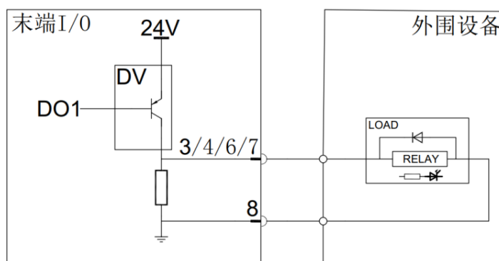
图 2-47: PNP 模式
