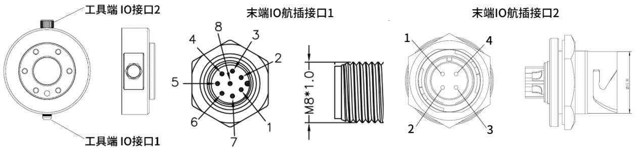
图 2-40: 机器人末端 I/O 航空插接口
