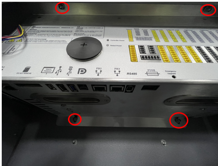
图 3-32: 螺母位置
