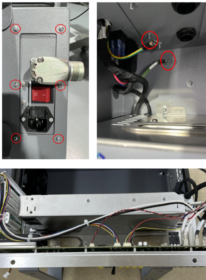
图 3-25: 螺钉位置、电源接地连接位置及钣金模块放置方式
