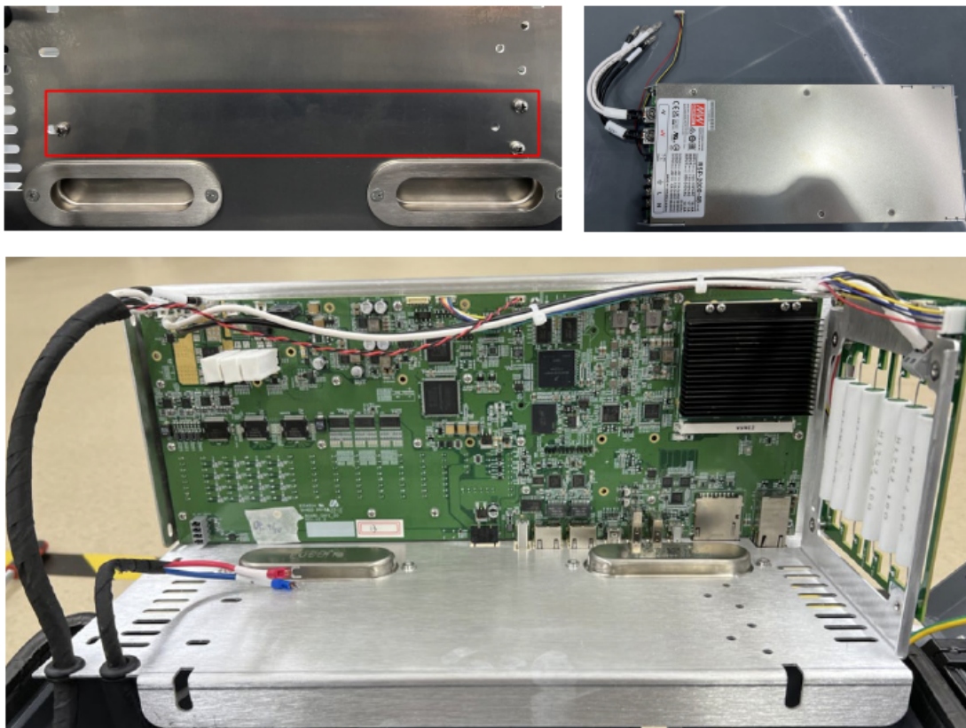
图 3-27: 螺钉位置及电源放置方式
