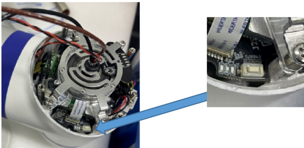
图 3-5: 白色按钮
