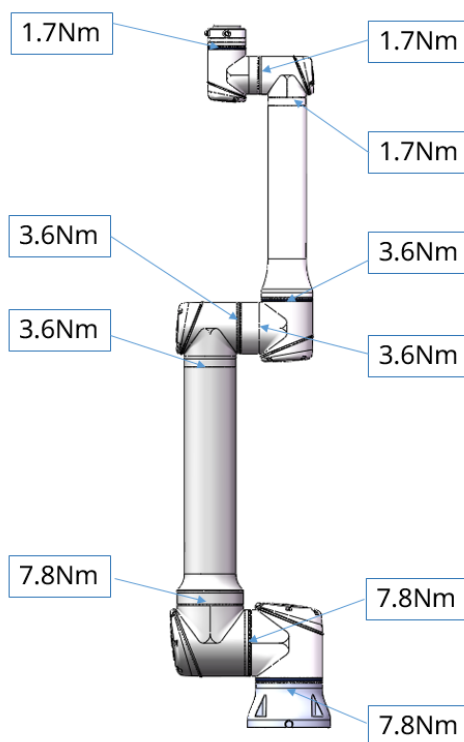
图 3-7: 各关节扭矩图
