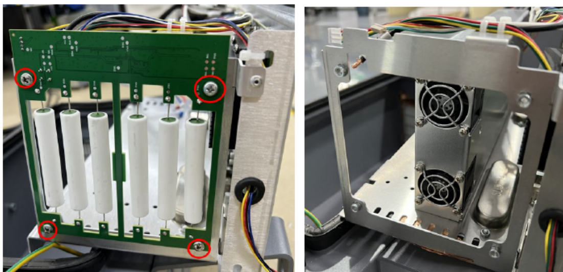
图 3-36: 取下刹车板
