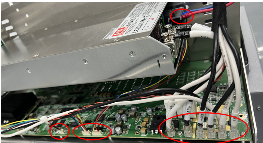
图 3-31: 线缆连接
