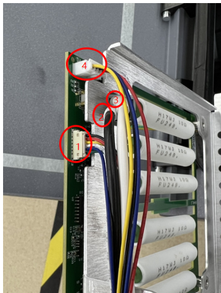
图 3-35: 断开线缆
