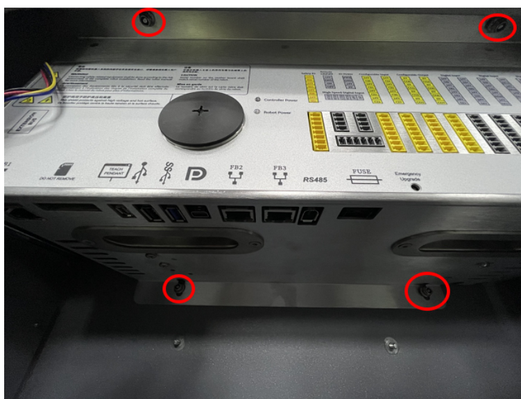
图 3-32: 螺母位置
