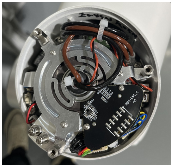
图 3-16: 重连电线
