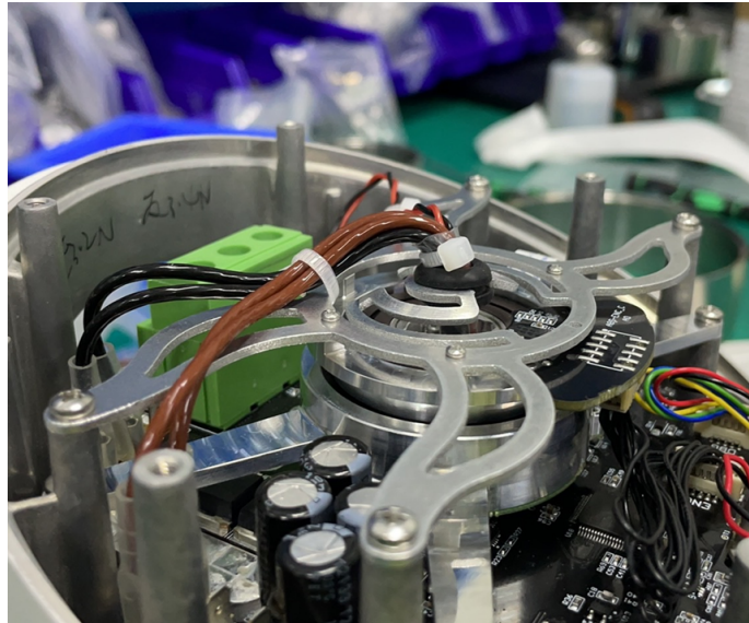
图 3-20: 接线和扎线
