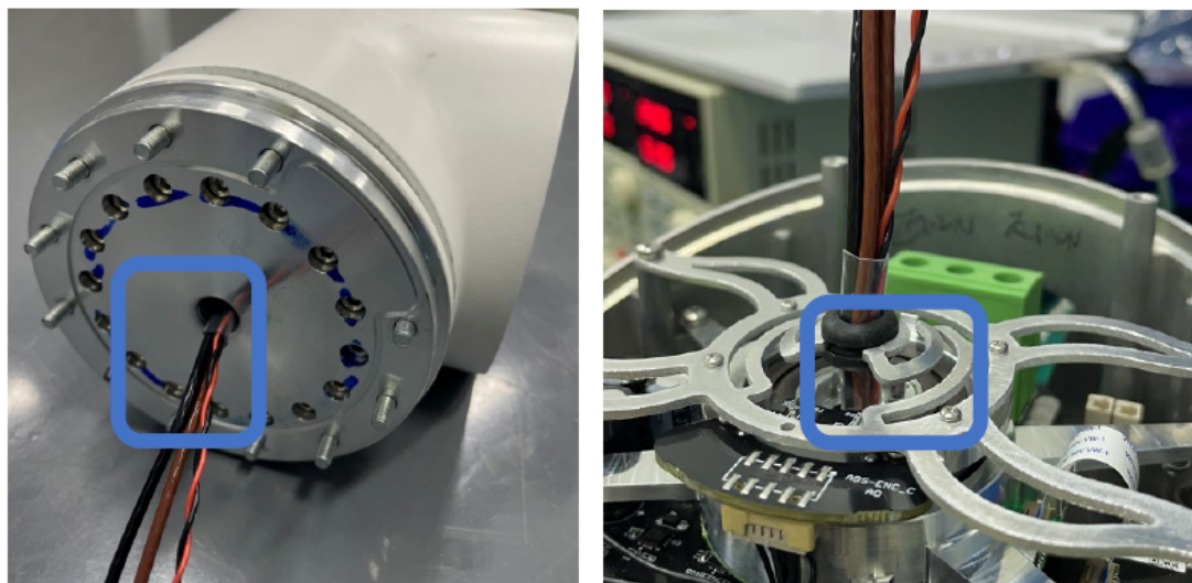
图 3-18: 线缆穿到关节上
