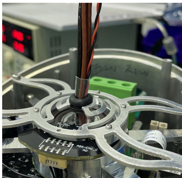
图 3-19: 套入护线环
