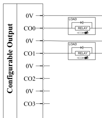
图 2-22: 配置输出接线方式
