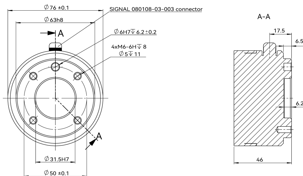
图 2-5: ES66 机器人工具法兰安装尺寸图，单位 mm
