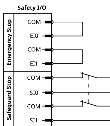
图 2-19: 控制柜的防护停止装置连接
