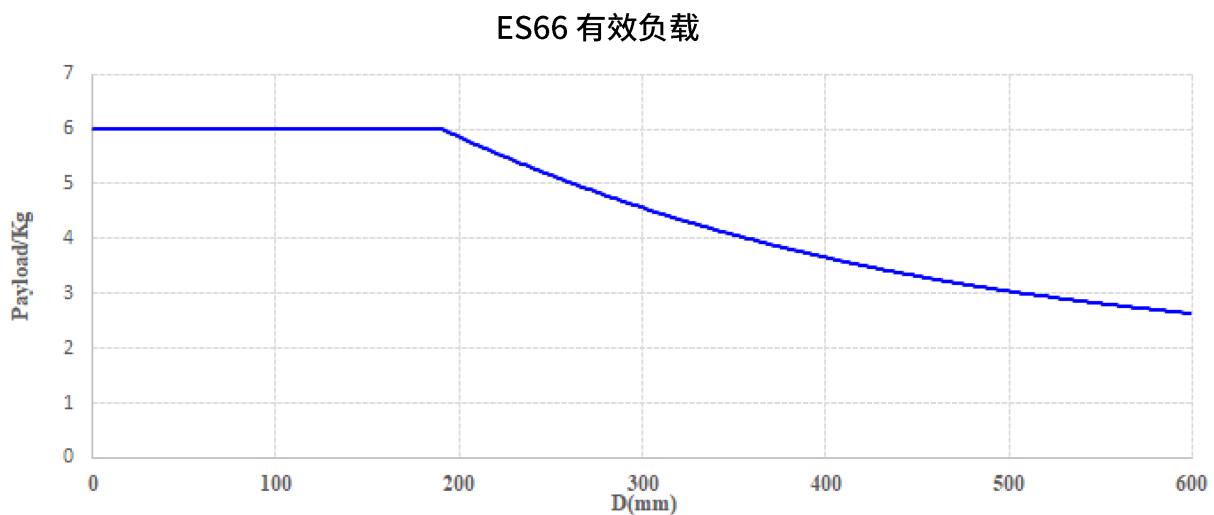
图 2-6: 有效负载图
