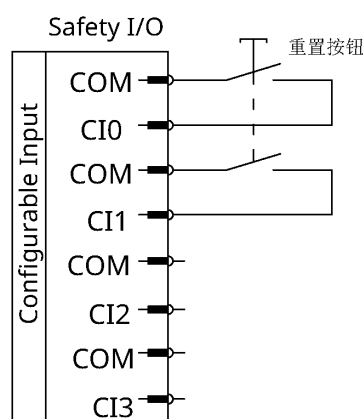
图 2-20: 控制柜的重置按钮连接方式
