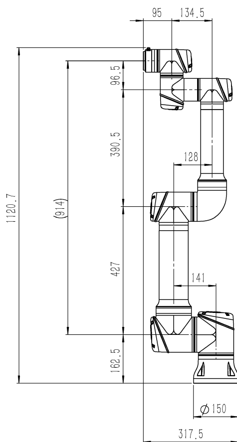
图 2-1: ES66 机器人机械尺寸图，单位 mm
