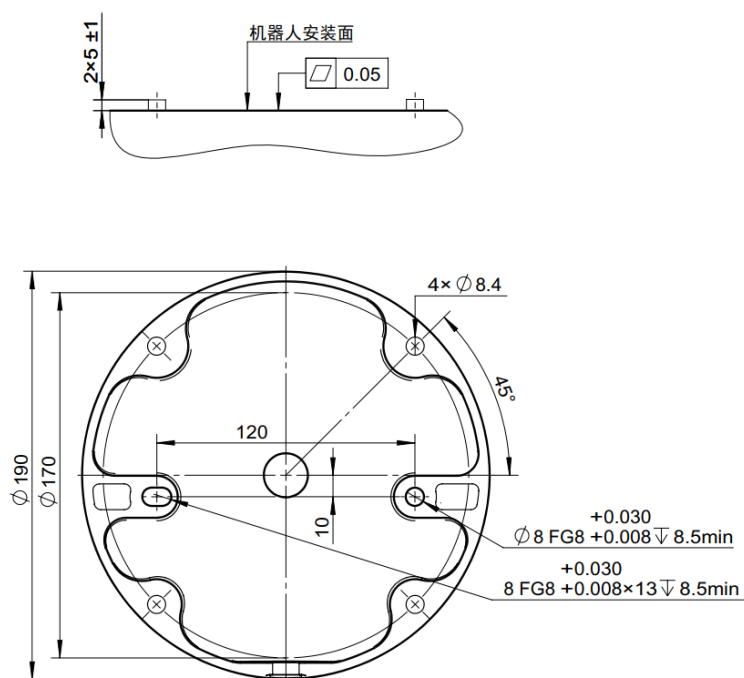
图 2-4: ES618 机器人基座安装尺寸图，单位 mm
