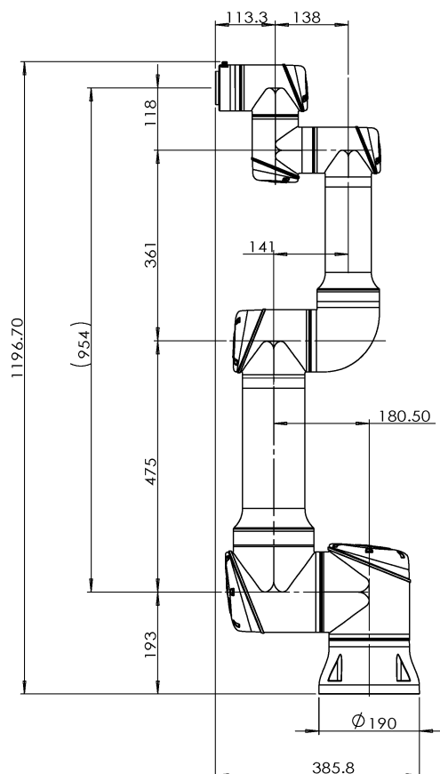
图 2-1: ES618 机器人机械尺寸图，单位 mm
