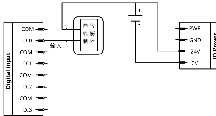
图 2-26: 数字输入 NPN 型接线（外部供电）
