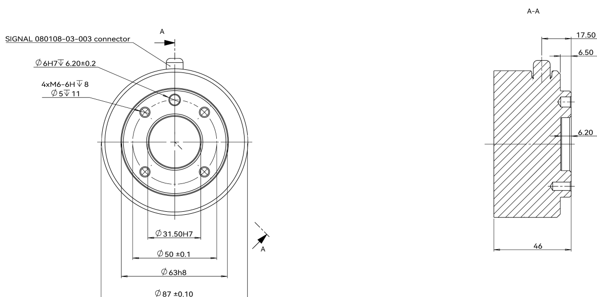
图 2-5: ES618 机器人工具法兰安装尺寸图，单位 mm
