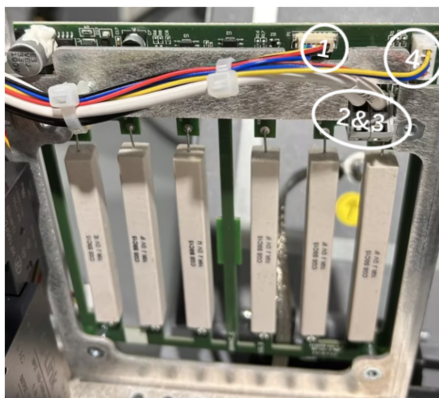
图 3-30: 断开线缆
