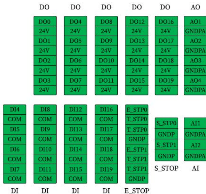
图 7-2：控制箱内部电气接口布局
