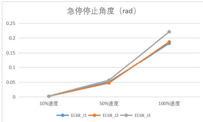
图 7-8 : EC68-08 急停停止
