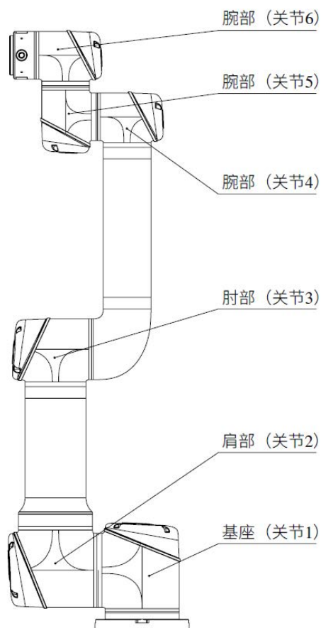
图 3-2：EC68-08 机器人关节
