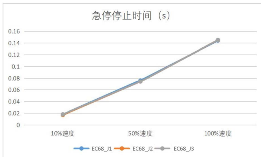
图 7-9 : EC68-08 急停停止时间
