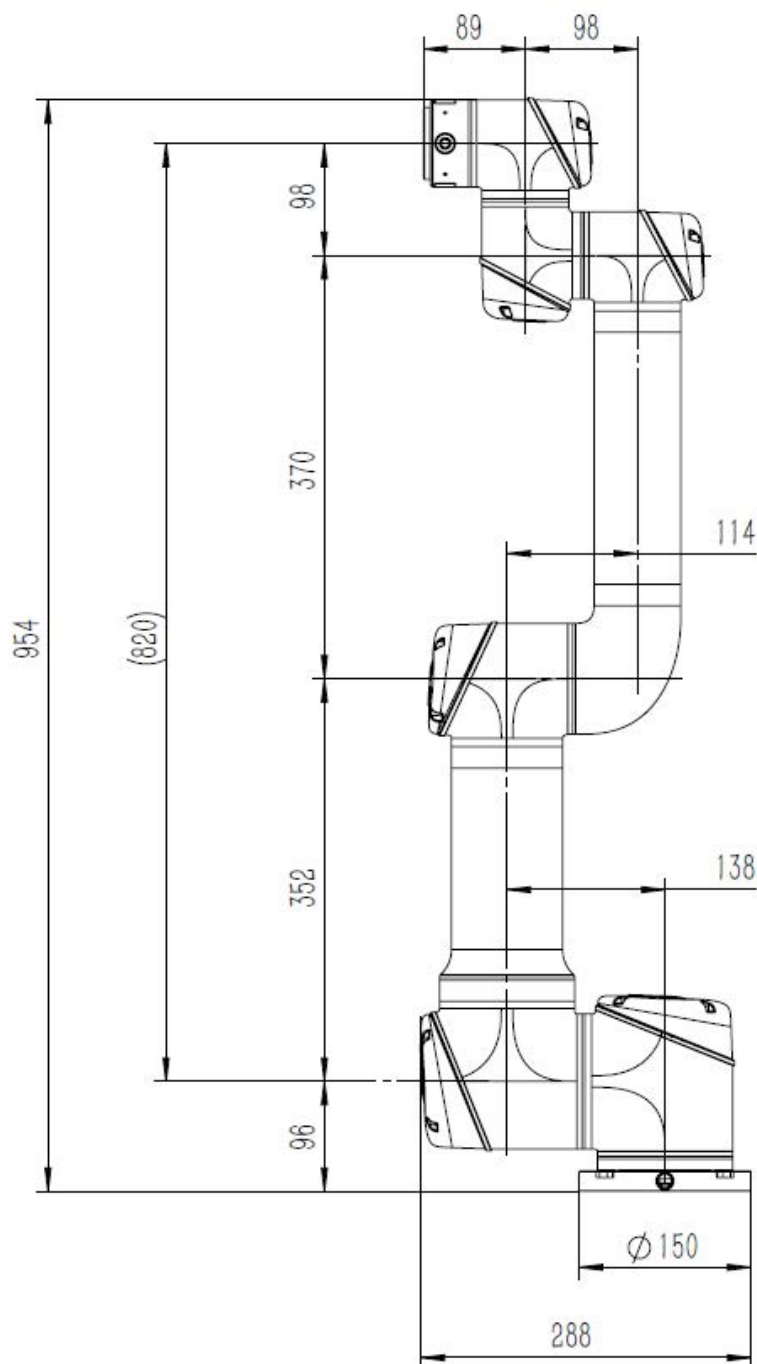
图 3-3：EC68-08 机器人的机械尺寸图，单位为 mm
