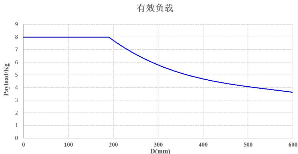
图 5-9：有效负载图
