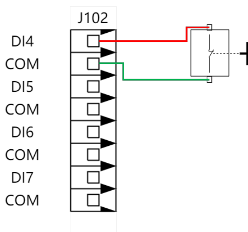
图 7-11：两线制传感器
