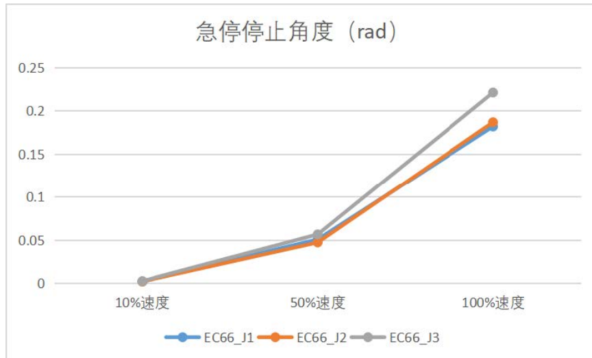
图 7-8 : EC66 急停停止角度
