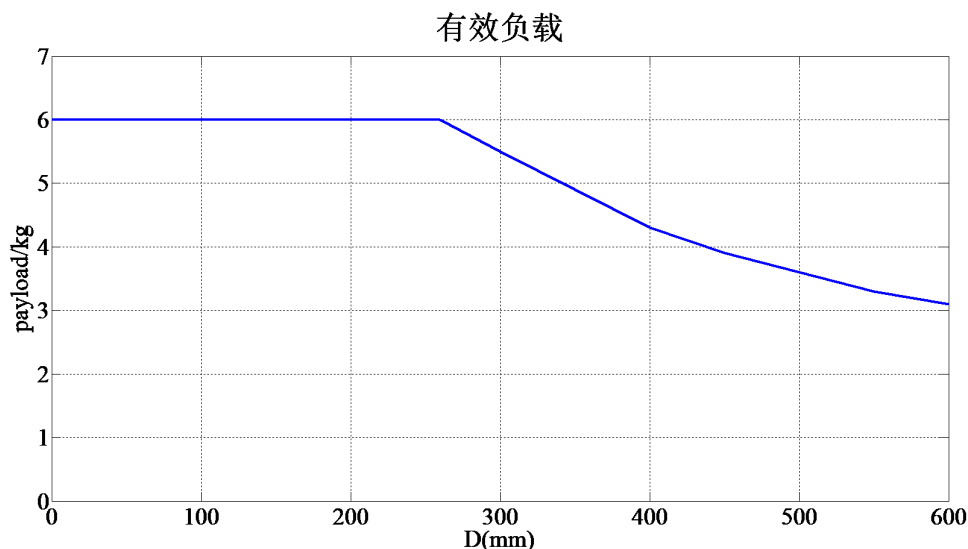
图 5-9：有效负载图
