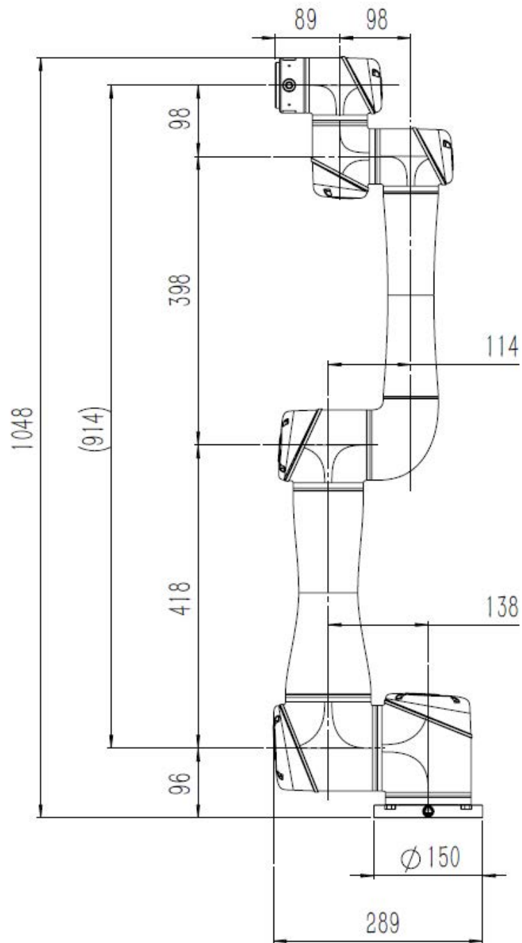
图 3-3：EC66 机器人的机械尺寸图，单位为 mm
