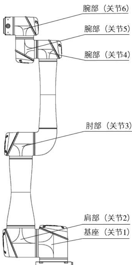
图 3-2：EC66 机器人关节
