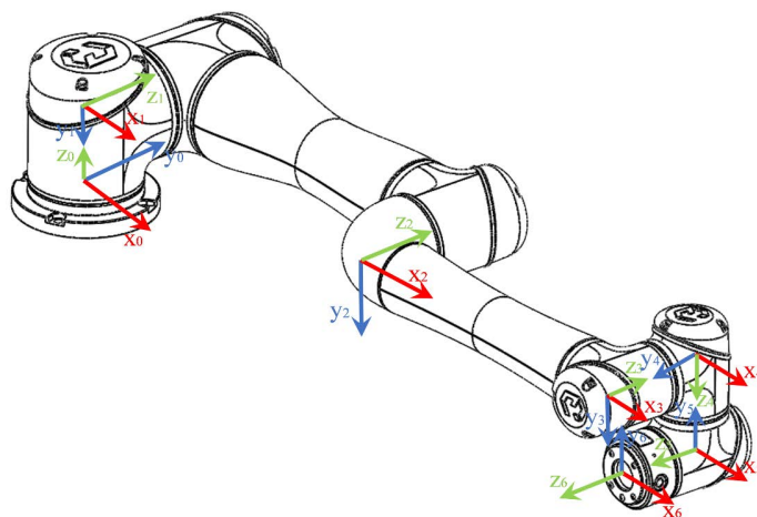
图 3-9 : 机器人 DH 示意图
