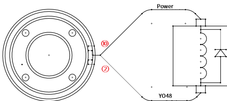
图 7-23：电感性负载
