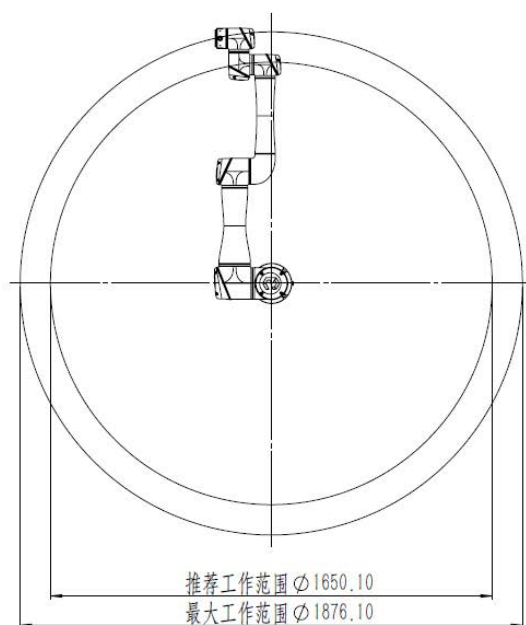
图 3-7：机器人工作空间俯视图
