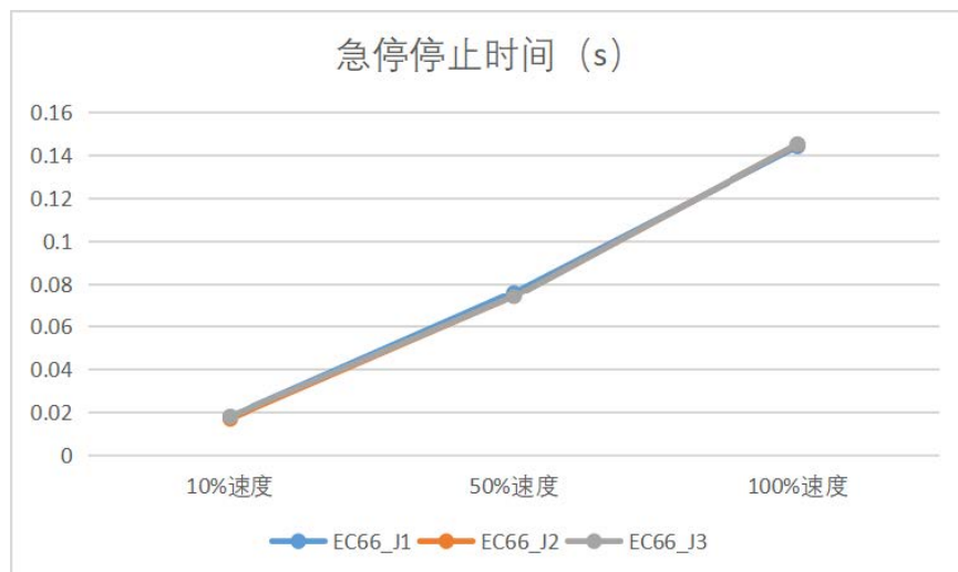
图 7-9 : EC66 急停停止时间
