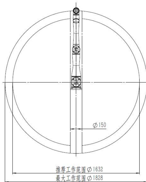
图 3-8：机器人工作空间侧视图
