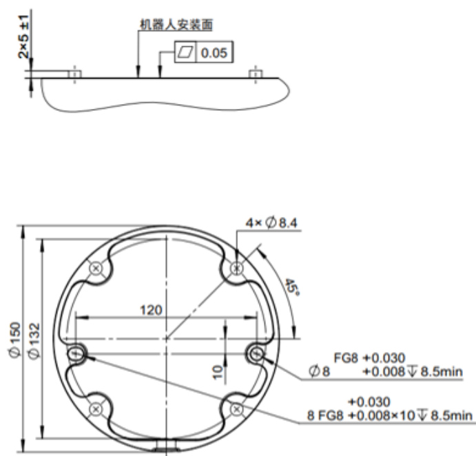
图 2-4: CS66 机器人基座安装尺寸图，单位 mm
