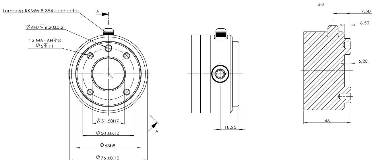
图 2-5: CS66 机器人工具法兰安装尺寸图，单位 mm
