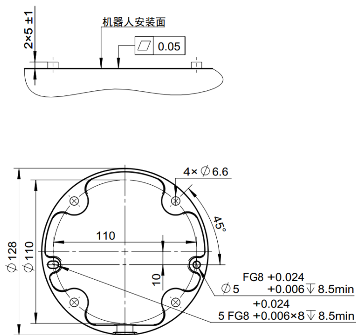
图 2-4: CS63 机器人基座安装尺寸图，单位 mm
