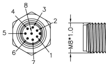
图 2-40: 机器人末端 I/O 航空插头接口
