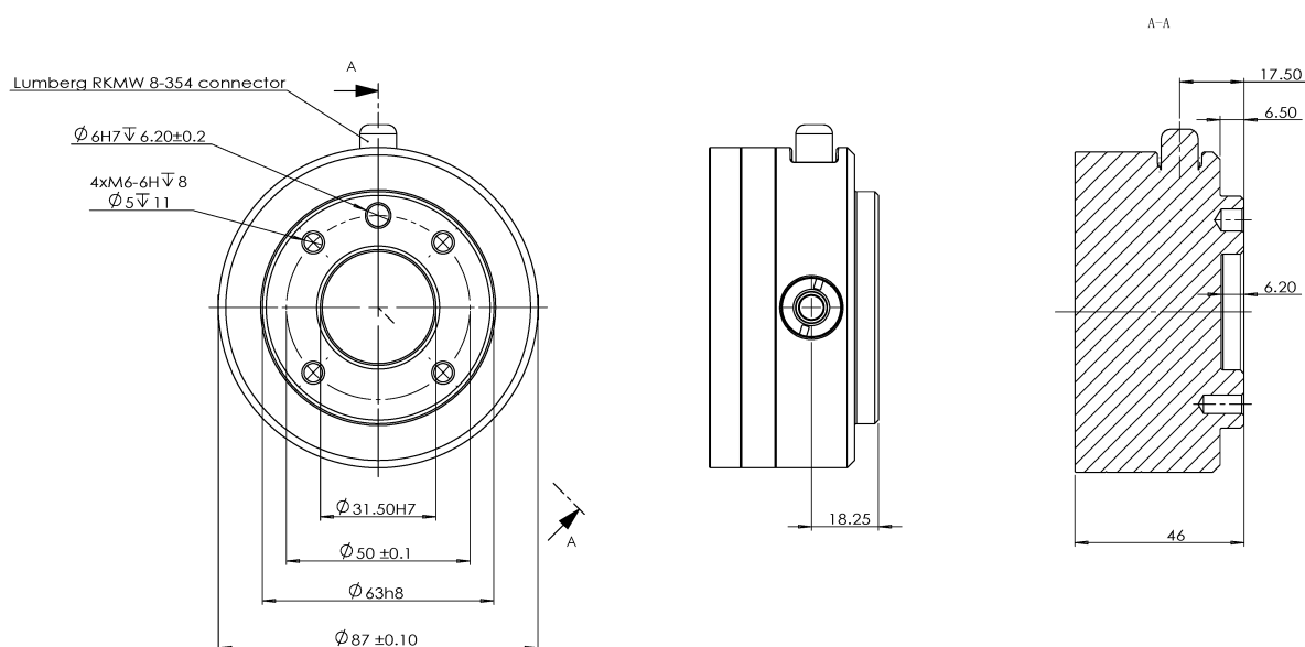
图 2-5: CS612 机器人工具法兰安装尺寸图, 单位 mm
