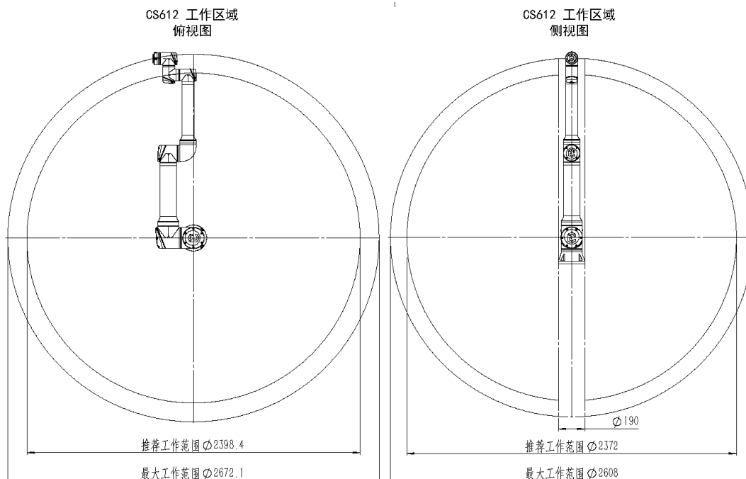
图 2-2: CS612 机器人工作空间, 单位 mm
