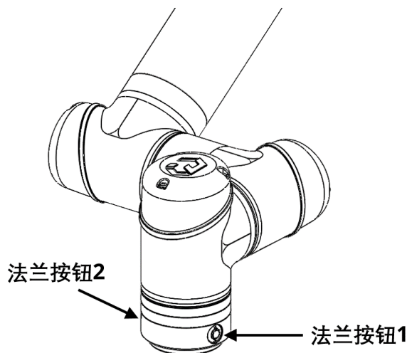
图 2-6: CS612 机器人末端法兰按钮
