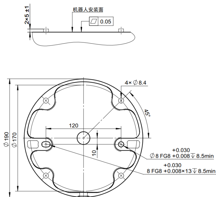
图 2-4: CS612 机器人基座安装尺寸图, 单位 mm
