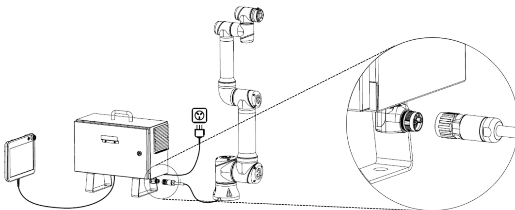
图 1-5: 整机安装-本体电缆未连接
