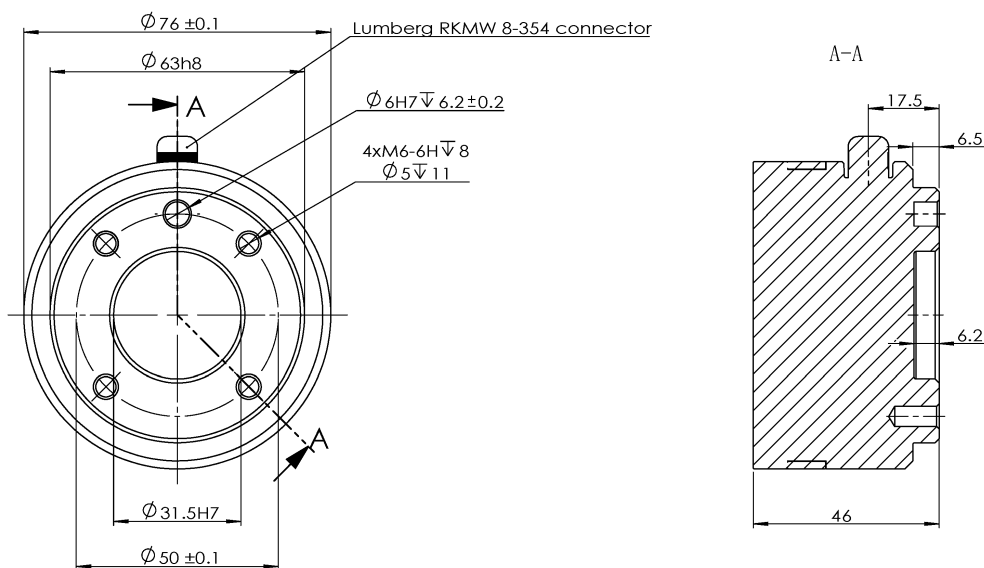
图 2-5: ES68 机器人工具法兰安装尺寸图，单位 mm
