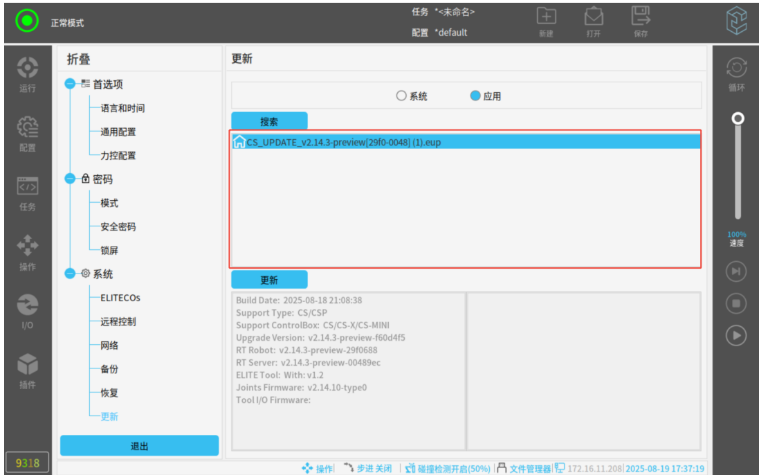
图 3-27: 应用更新
