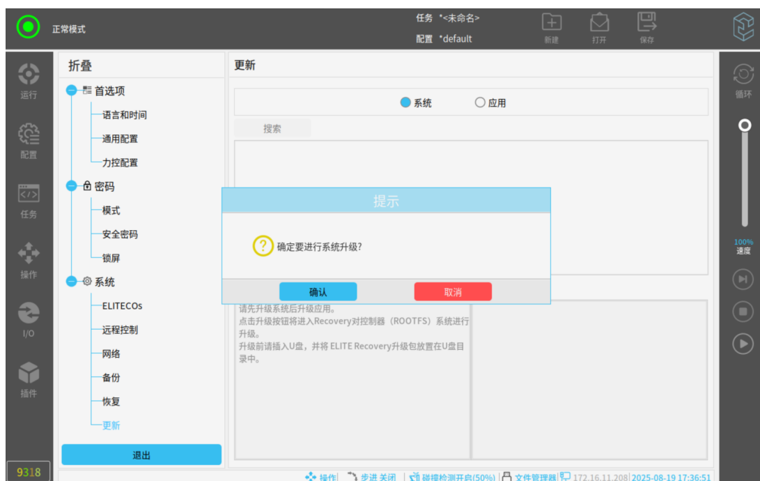
图 3-26: 系统更新
