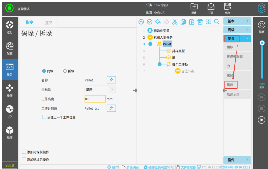
图 3-122: 设置码垛任务参数
