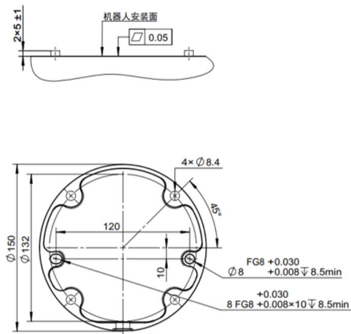
图 2-4: ES68 机器人基座安装尺寸图，单位 mm
