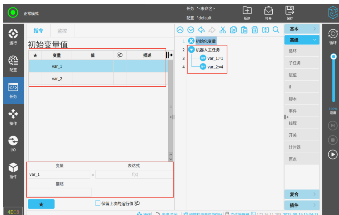
图 3-80: 可选的变量
