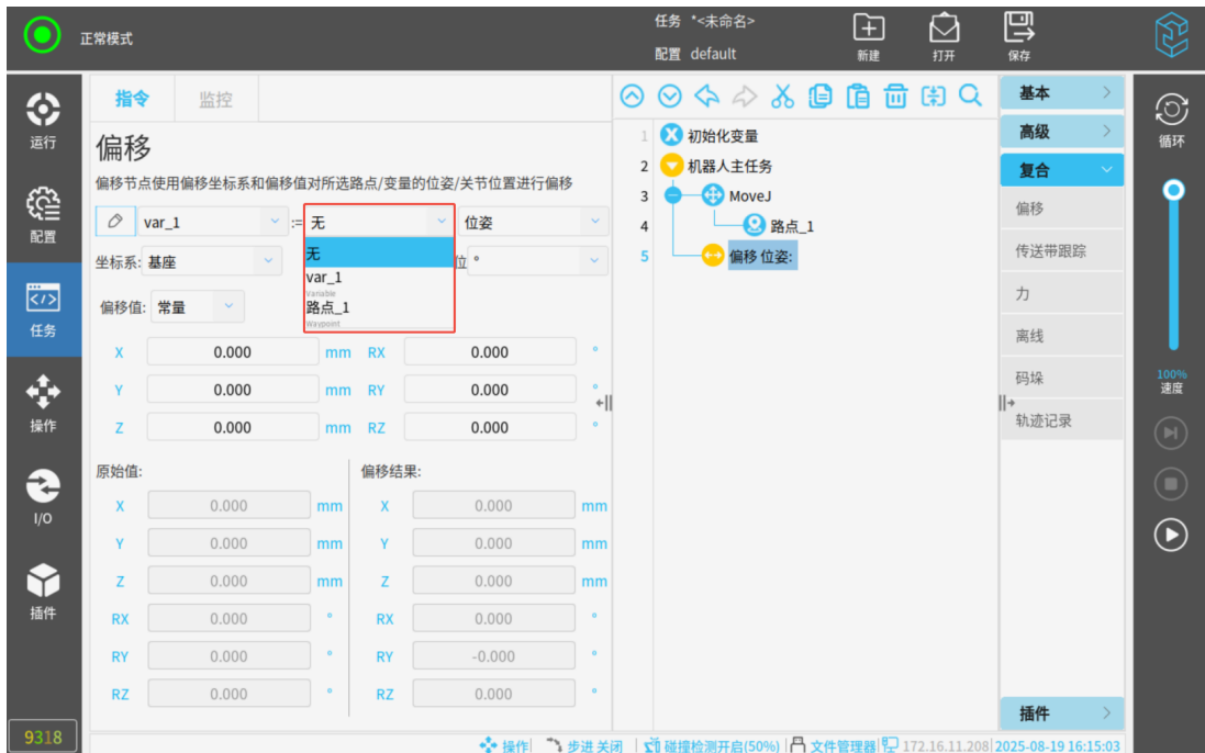
图 3-110: 选择数据源
