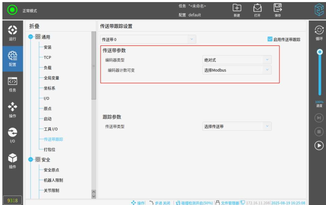
图 3-126: 配置传送带参数
