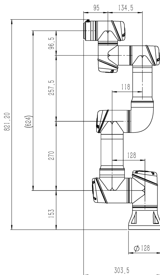
图 2-1: ES63 机器人机械尺寸图，单位 mm
