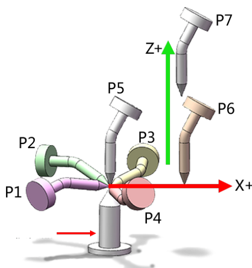
图 3-40: 三点法示教坐标系方向
