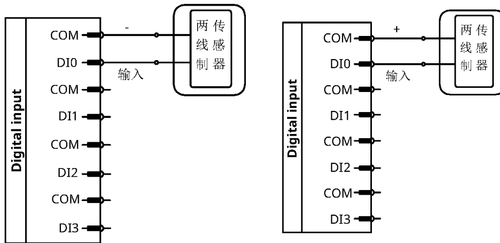
图 2-23: 数字输入 NPN 型接线 (内部供电) 图 2-24: 数字输入 PNP 型接线 (内部供电)
