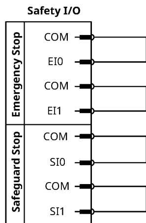
图 2-17: 安全 I/O 默认配置连接
