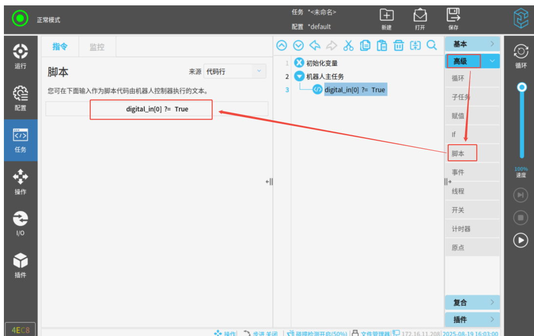
图 3-102: 脚本
