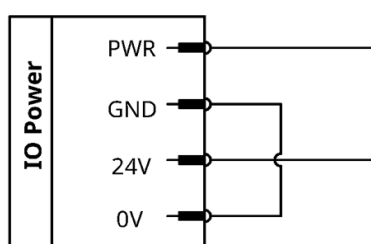
图 2-32: 使用内部电源接线方式
