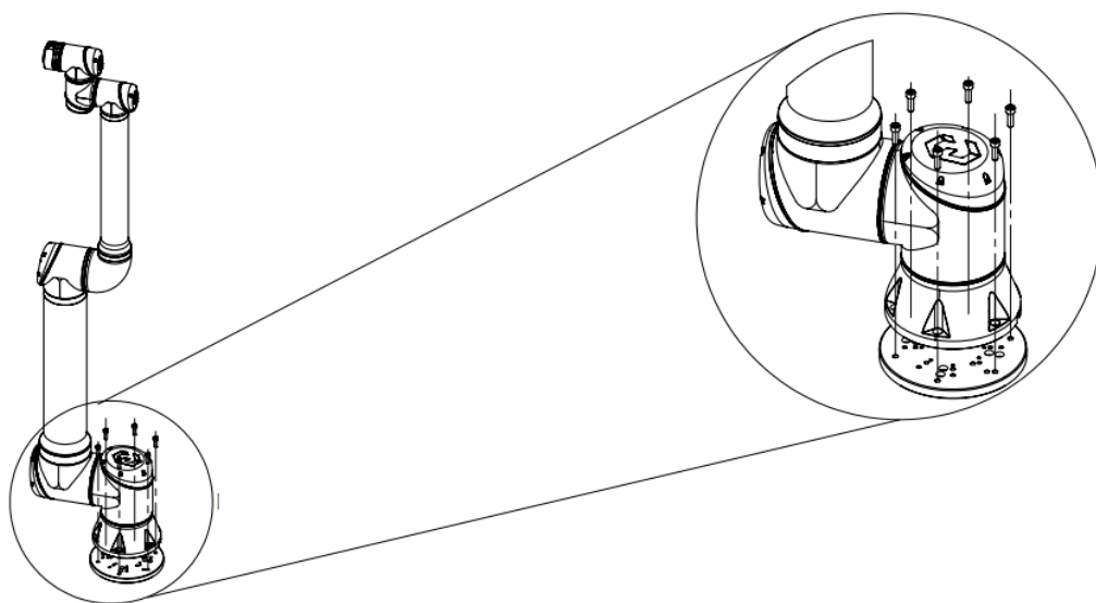
图 1-3: 本体安装
