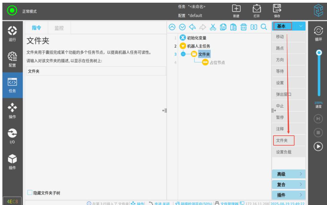
图 3-96: 文件夹
