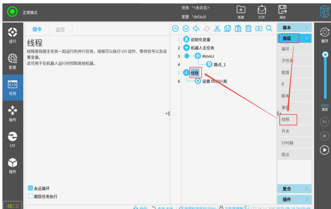
图 3-104: 线程
