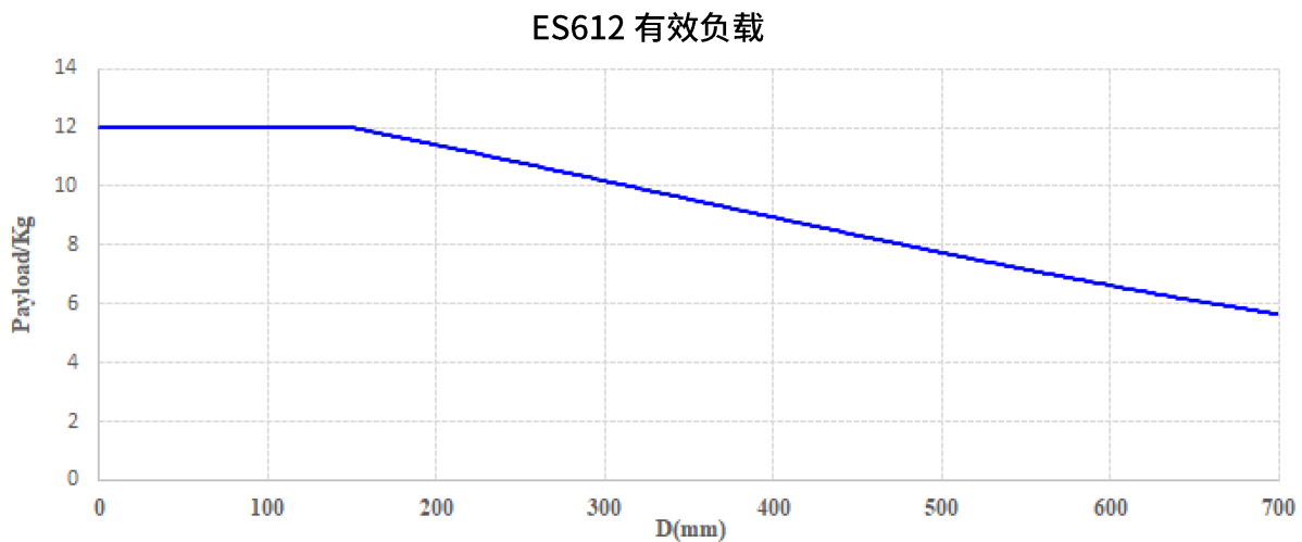
图 2-6: 有效负载图
