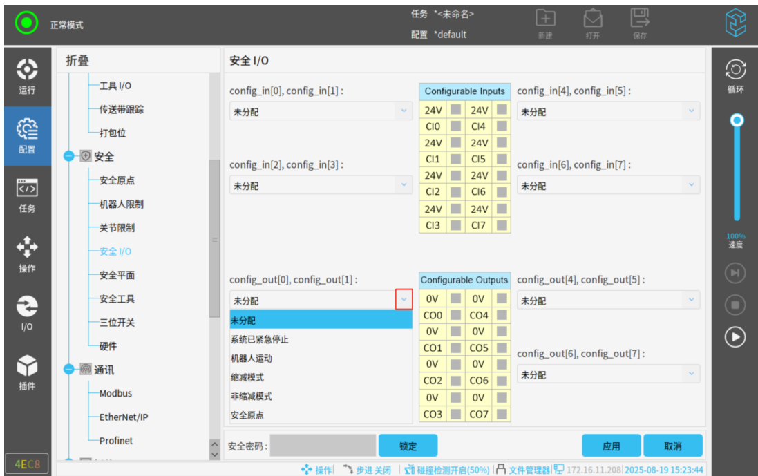
图 3-66: 输出信号
