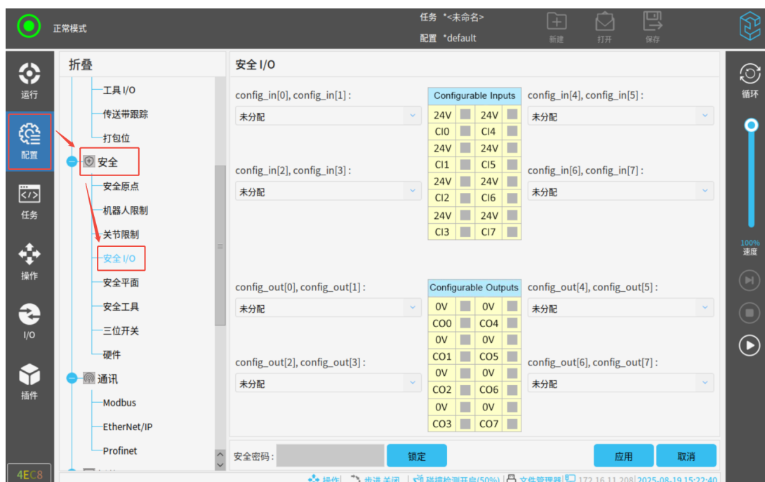
图 3-64: 安全 I/O
