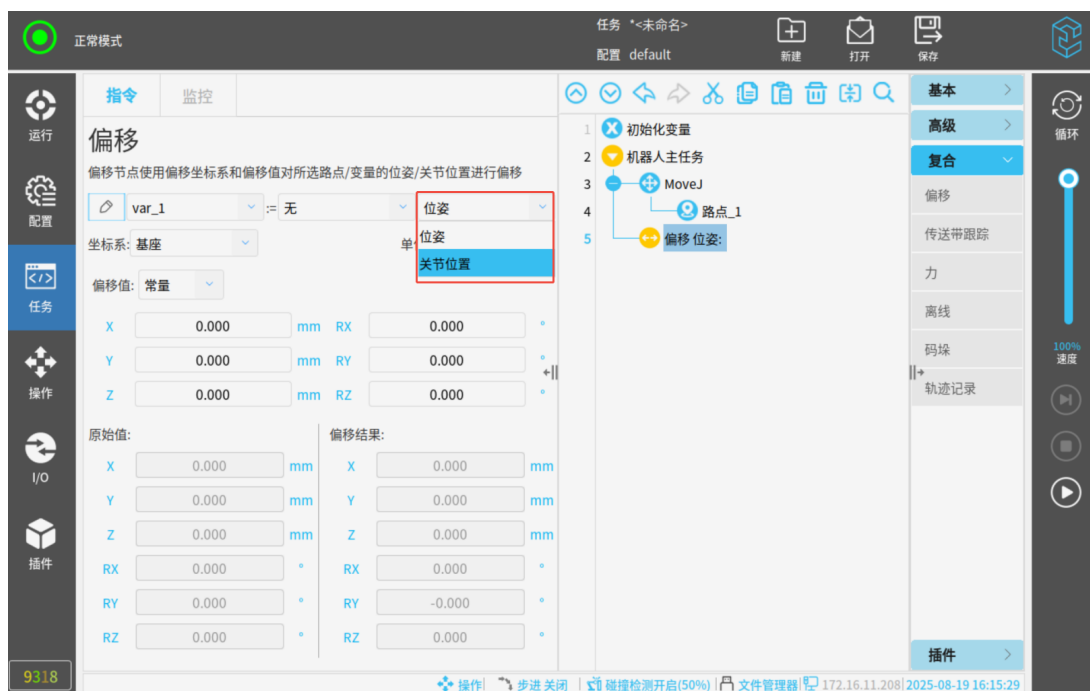
图 3-111: 选择路点的引用数据类型
