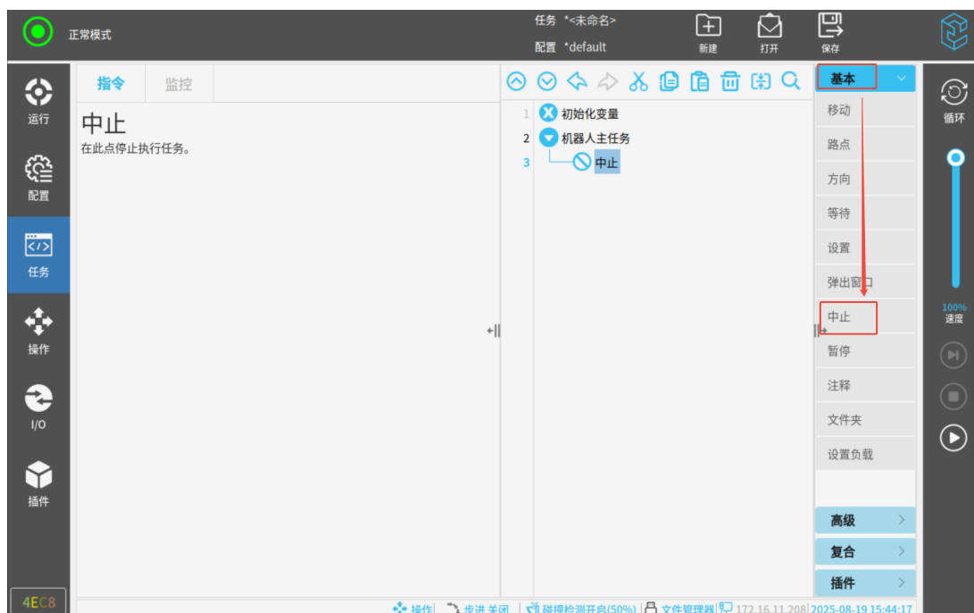
图 3-93: 中止
