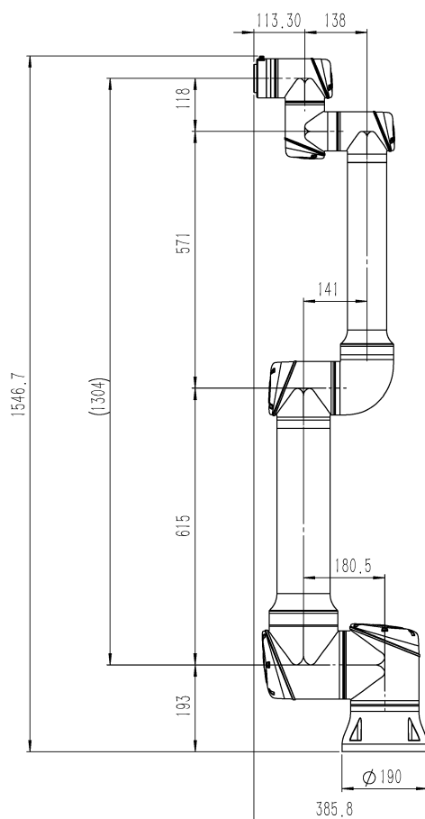
图 2-1: ES612 机器人机械尺寸图，单位 mm
