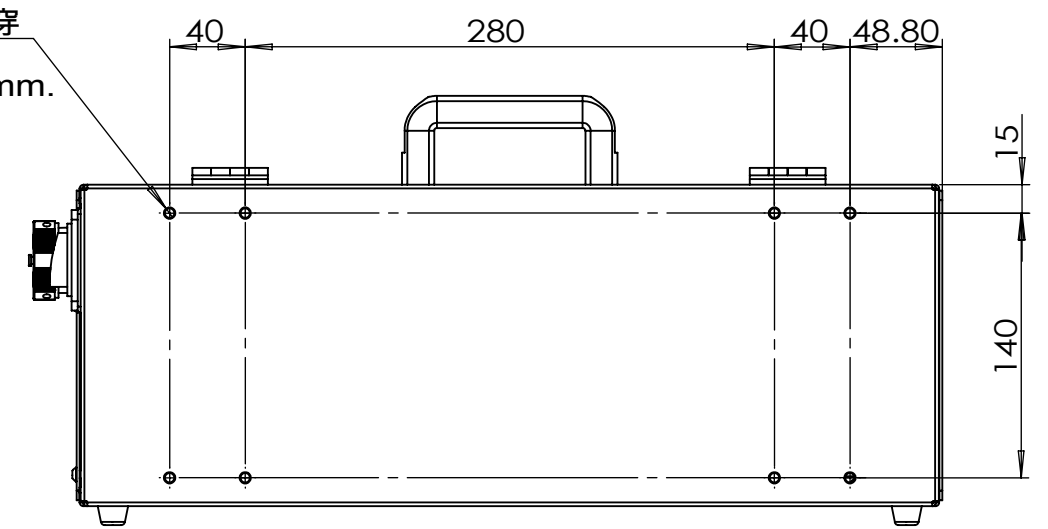
后视图
