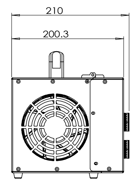
后视图
